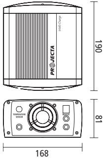
IC800-24
